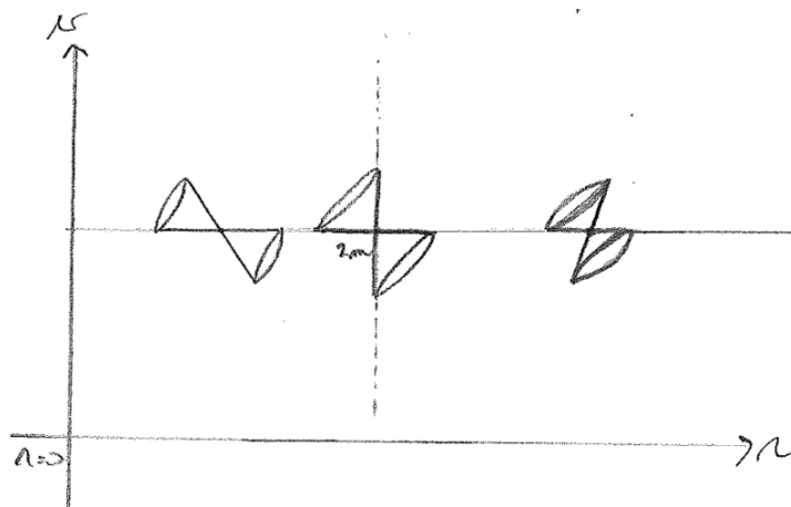
FIGURE 8.5 – Les cônes de lumière dans les coordonnées d'Eddington-Finkelstein entrantes. La ligne horizontale v = \text{cte} correspond aux rayons lumineux entrants, donc le bord du cône de lumière.
